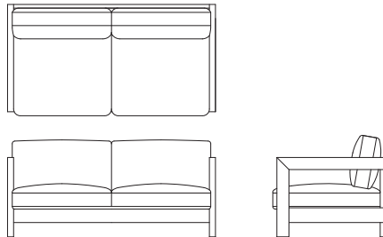
ワイド2Pソファ L08710F [W/1545 D/830 H/760 SH/400] OIL WN
